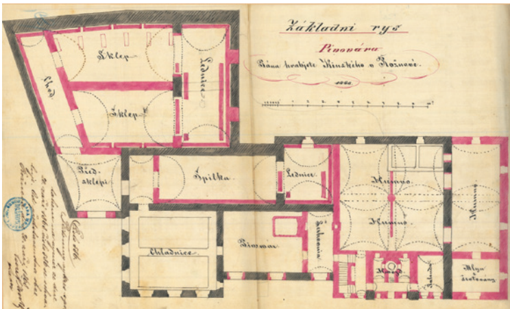
Základní rys pivovaru z roku 1868.
